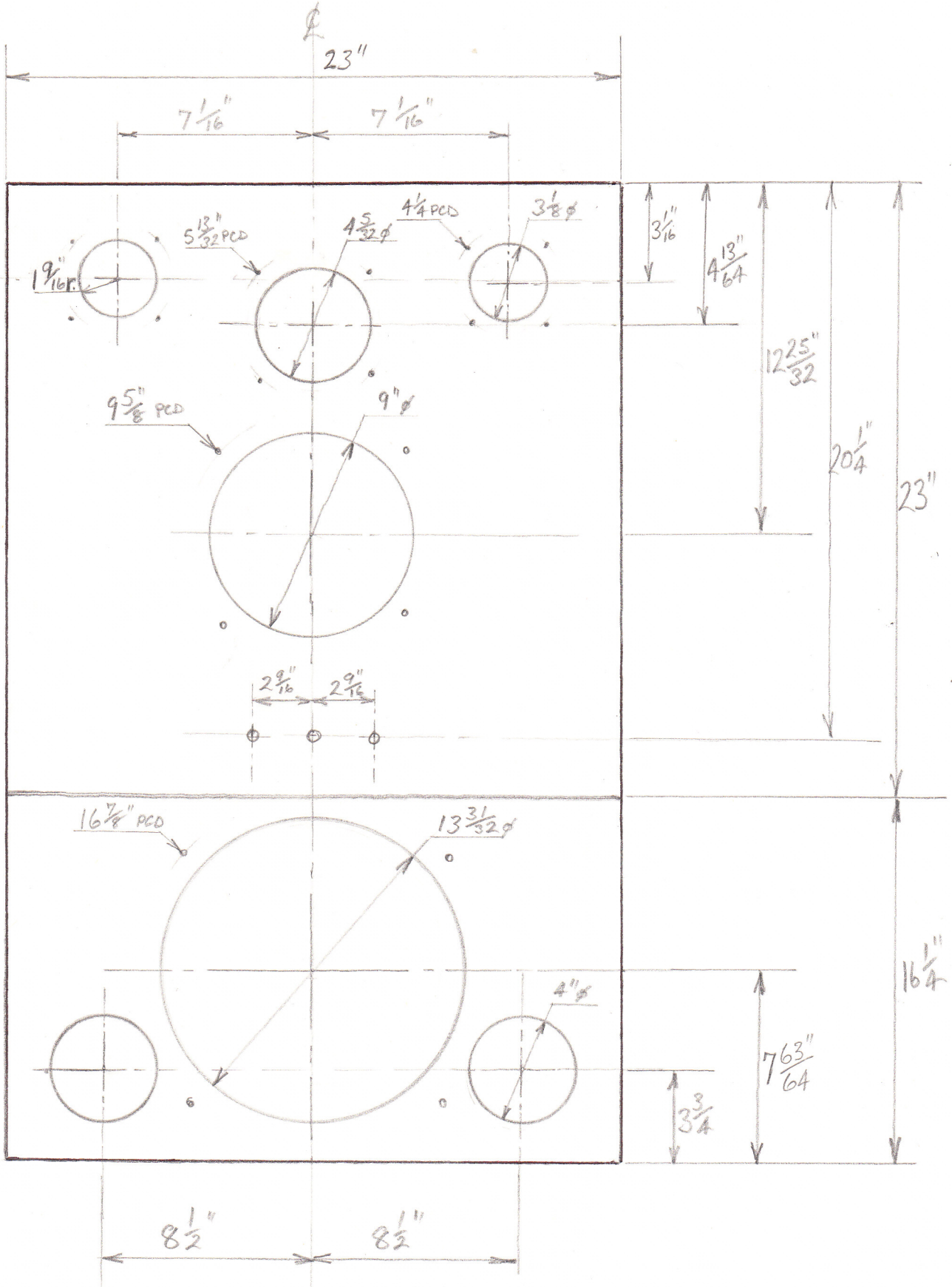
JBL 4343 Baffle Layout
